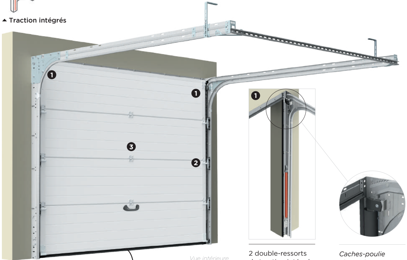
Vue intérieure
