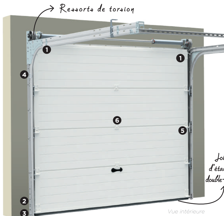
▲ Traction intégrés
